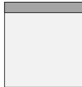
図 1 起動画面
